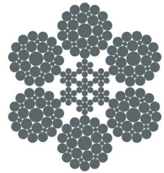
6×29F-IWRC
