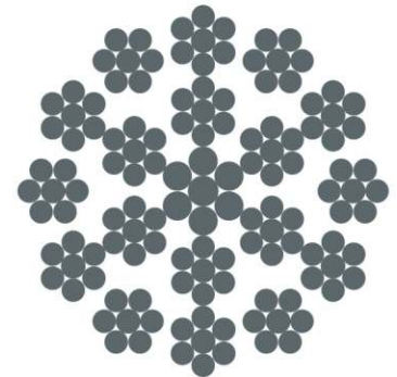
18×7-WSC
