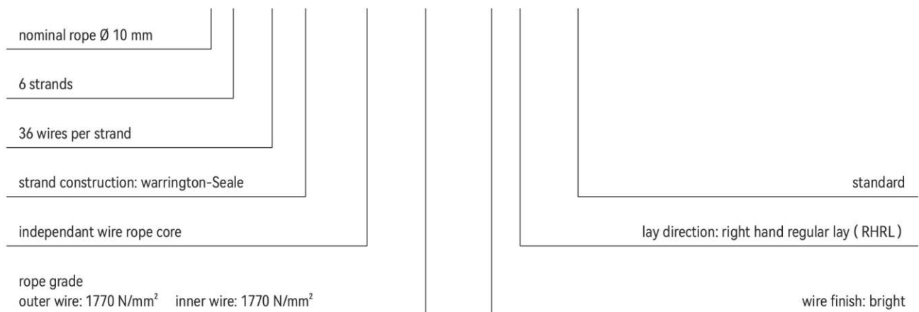
6×36WS-IWRC
