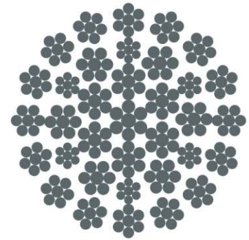
35(W)×7
