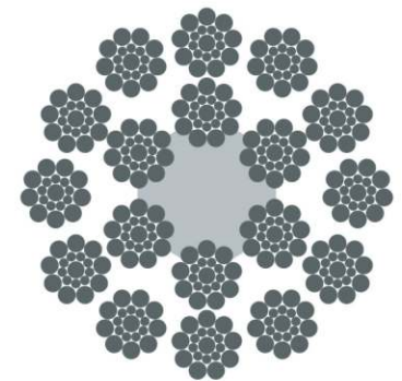
18×19S-FC
