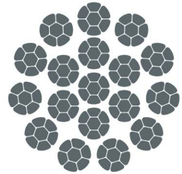
17xK7-WSC
