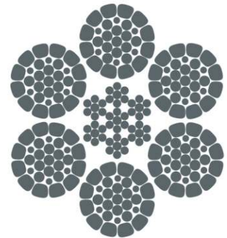
6×K31WS-IWRC
