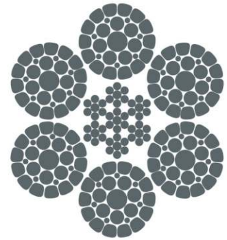
6×K29F-IWRC
