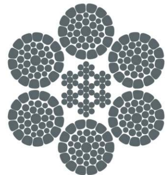
6×K36WS-IWRC
