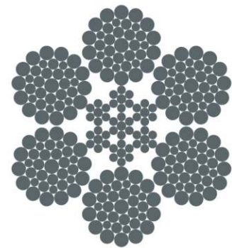
6×36WS-IWRC
