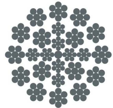
24(W)×7
