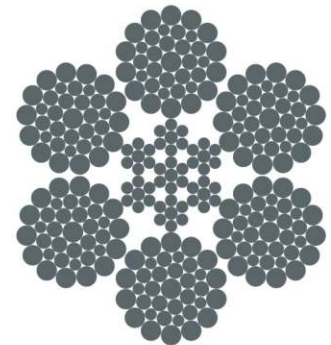
6×36WS-IWRC
