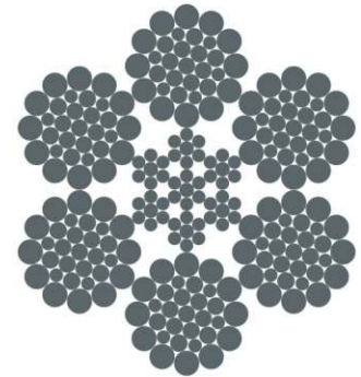
6×31WS-IWRC
