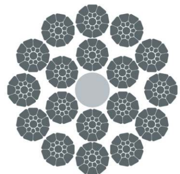
18×K19S-FC
