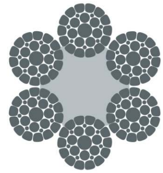
6×K29F-FC
