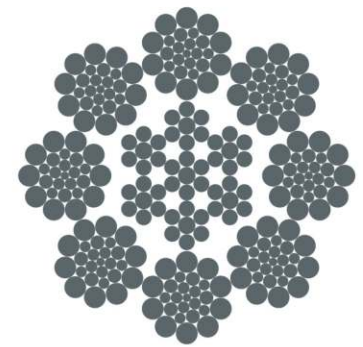
8×26WS-IWRC
