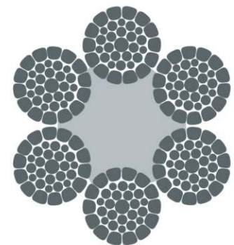
6×K36WS-FC
