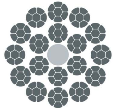
18×K7-FC
