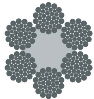
6×36WS-FC
