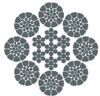
8×K26WS-IWRC(7x7)
